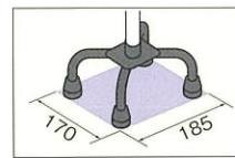
スモールベース 重量 785g
