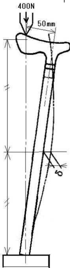
図4 圧縮試験
